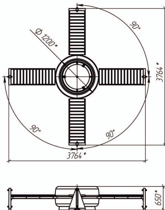
Исполнение -03
