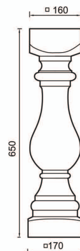
АФБ 04 - 08 балясина
