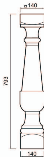
АФБ 04 - 03 балясина
