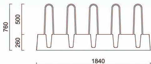
велопарковка АФБ 06 - 03
