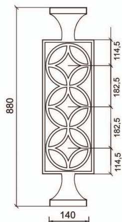
АФБ 04 - 01 балясина
