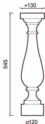
АФБ 04 - 06 балясина
