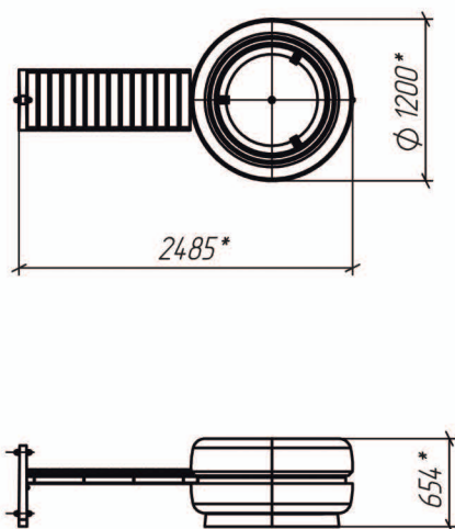
Исполнение -00
