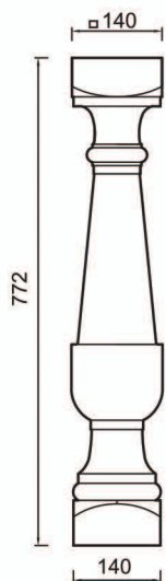
АФБ 04 - 02 балясина
