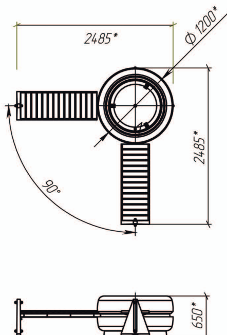
Исполнение -01
