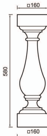
АФБ 04-07 балясина
