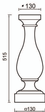
АФБ 04 - 05 балясина
